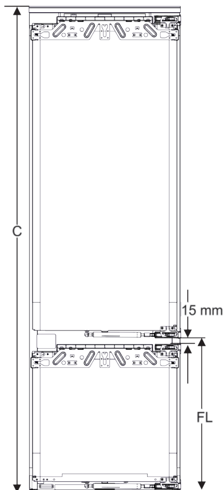
Fig. 67 Положение зазора двухдверного мебельного фасада
